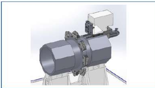
UNITÀ MONOASSE
